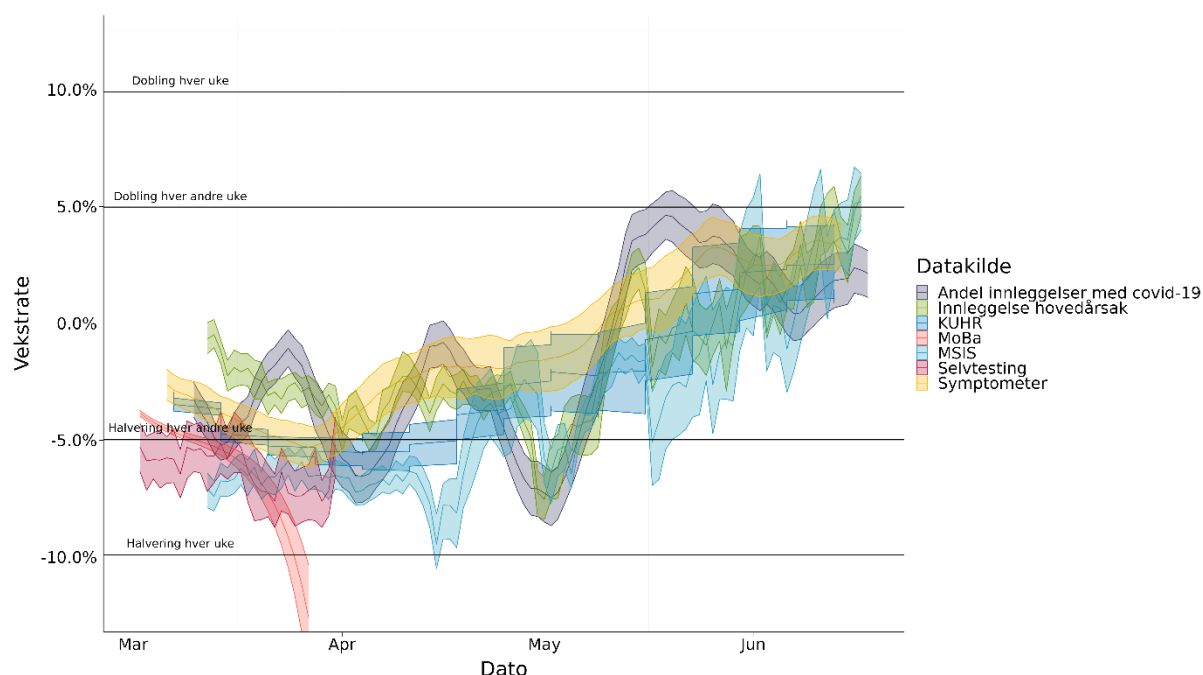
Figur 21. Estimert vekstrate for nye smittede fra ulike datakilder. En positiv vekstrate indikerer en voksende epidemi og en negativ vekstrate en synkende epidemi. Alle datakildene har styrker og svakheter og må tolkes med varsomhet 20. november 2021– 21. juni 2022. Kilde: BeredtC19; NoPaR og NPR, MSIS, sKHUR, Symptometer, MoBa, Folkehelseinstituttet og selvtester fra kommunene via Helsedirektoratet.
